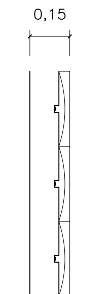
sezione parete
